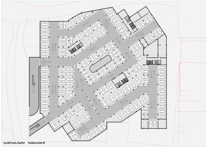
Նկար 4.1. Ստորգետնյա ավտոկանգառի հատակագիծ՝ 153 ավտոտեղ (բնակարանների քանակի 80%):
